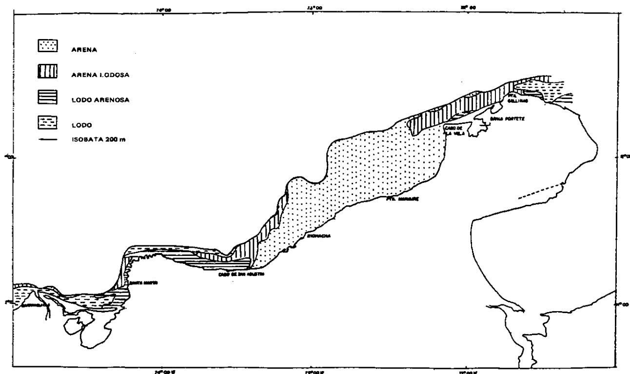
Figura 3. Distribución de los tipos de sedimentos presentes en la plataforma continental al noroeste del Caribe colombiano (modificado a partir de Javelaud, 1984 y Cuignon, 1985).
