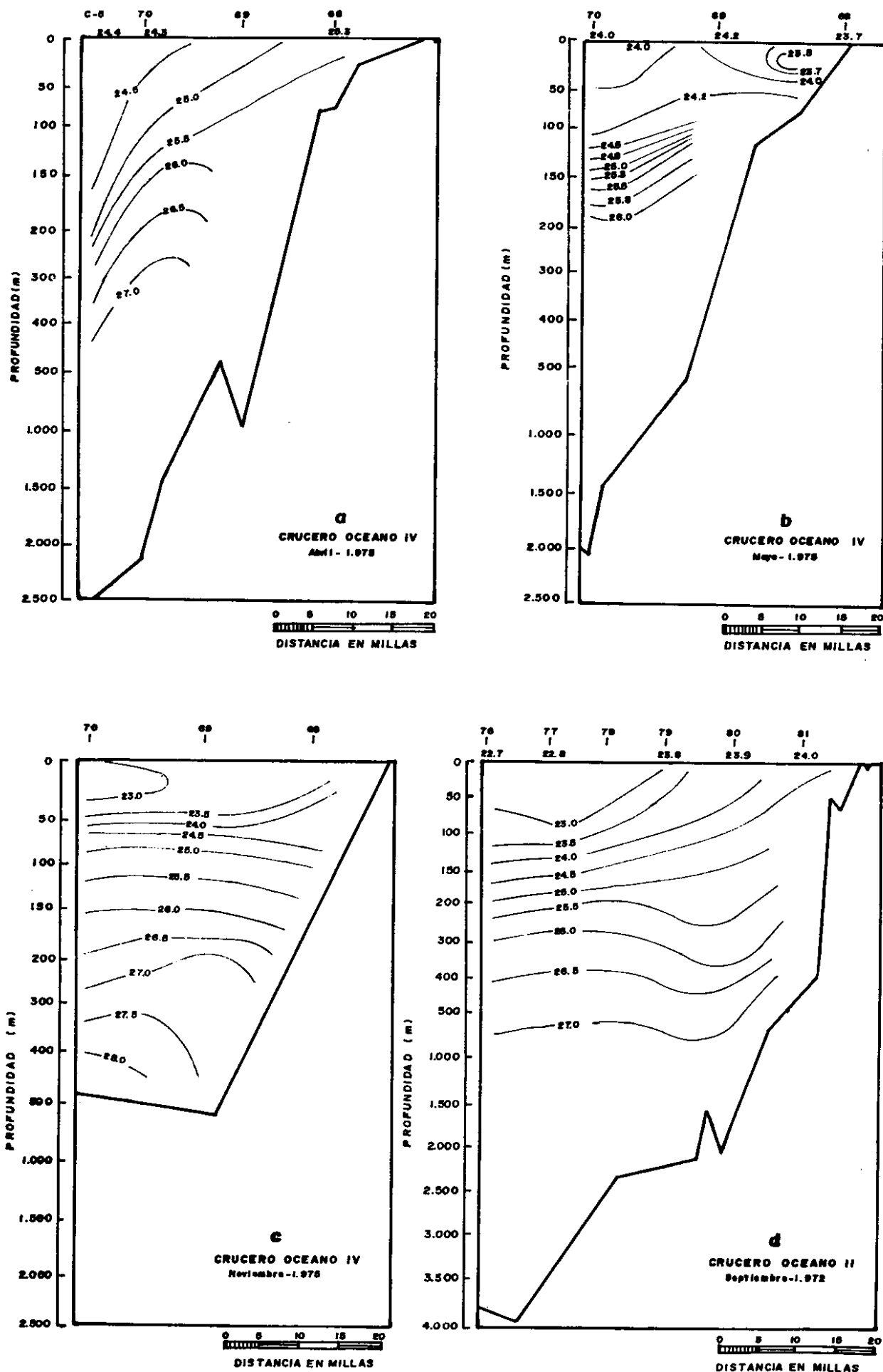
Figura 14. Distribución vertical del sigma-T ( T_t ) en los transectos 68-C5 y 76-81 de las campañas de abril, mayo, noviembre, (OCEANO IX de 1975) y de septiembre (OCEANO II de 1972), a bordo del B/O San Andrés.
