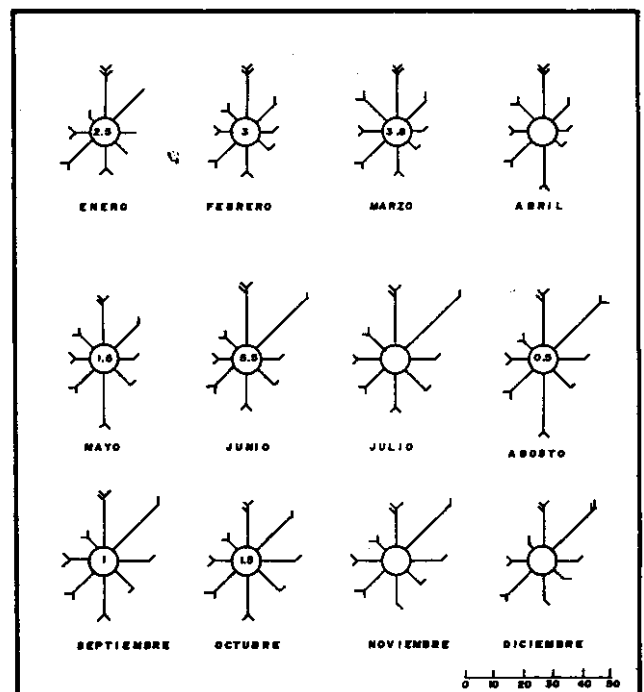
Figura 7. Regimen de vientos en el área de estudio, utilizando la escala de Beaufort, con base en los datos de los aeropuertos (a) Almirante Padilla de Riohacha (Gua.), y (b) Simón Bolívar de Santa Marta (Mag.), para 1981-1983 (HIMAT, com. pers).
