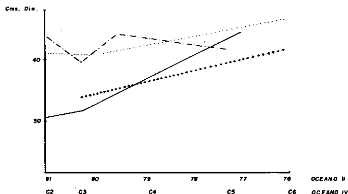
Figura 15. Altura del nivel del mar con referencia a 150 db para cuatro épocas diferentes: septiembre-octubre de 1972 (....), marzo (+++), abril (---) y noviembre (---) de 1975 (C2-C6, OCEANO II) (transectos 76-81, OCEANO IV), a bordo del B/O San Andrés.
