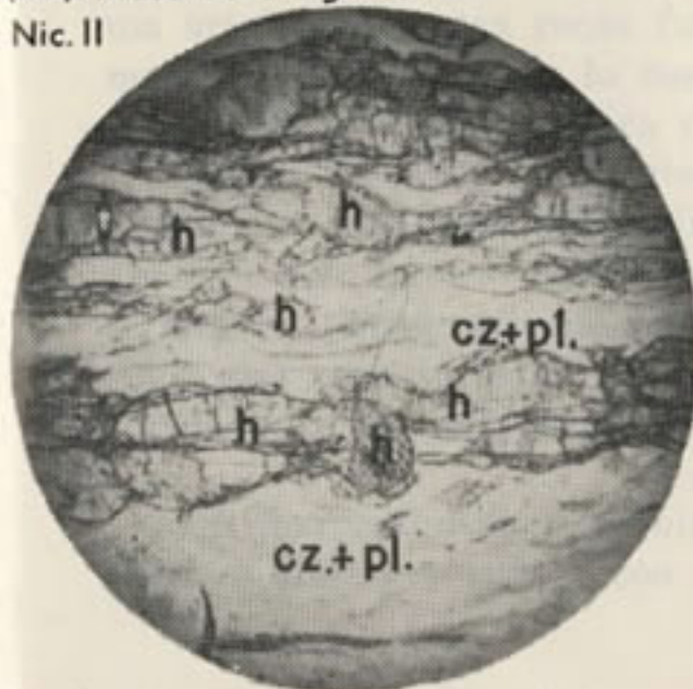
Fig.5-Contacto Serpentinita - Anfibolita. Roca N° 658-A. Efectos cataclásticos del contacto en cuarzo, plagioclasa (cz.+ pl.) y hornblenda (h.).
