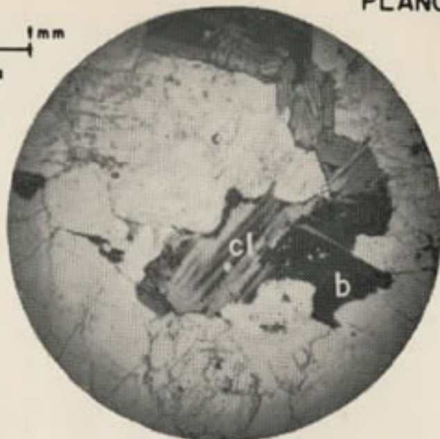
Fig.2- Batolito Antioqueño. Roca N° 746-A. Biotita (b) en proceso de cloritización. (cl.) Nic II
