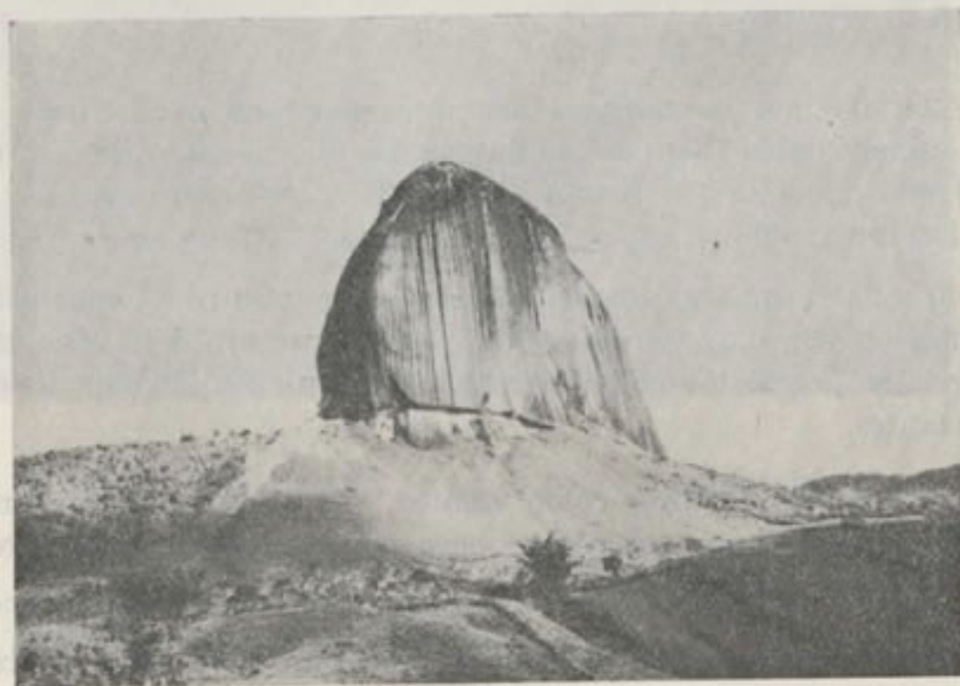
Fig. 7 - Peñol de Guatapé visto del Oeste
