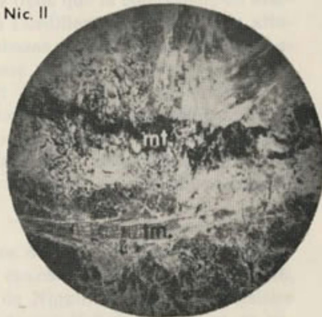
Fig.4- Serpentinita, Roca N° 314-A. Tremolita (tm.) magnetita (mt.) relleno de fisura. Masa de antigorita.
