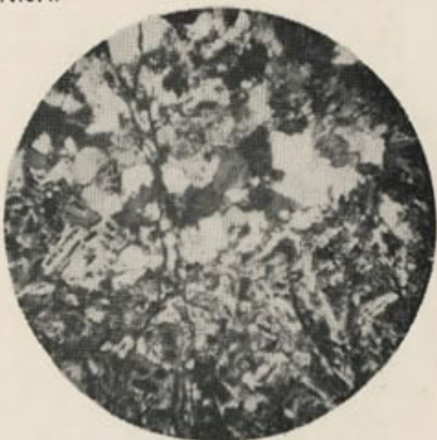
Fig. 6- Batolito de Altavista. Roca N° 1049-A Roca del contacto con anfíbolitas. Nic. +
