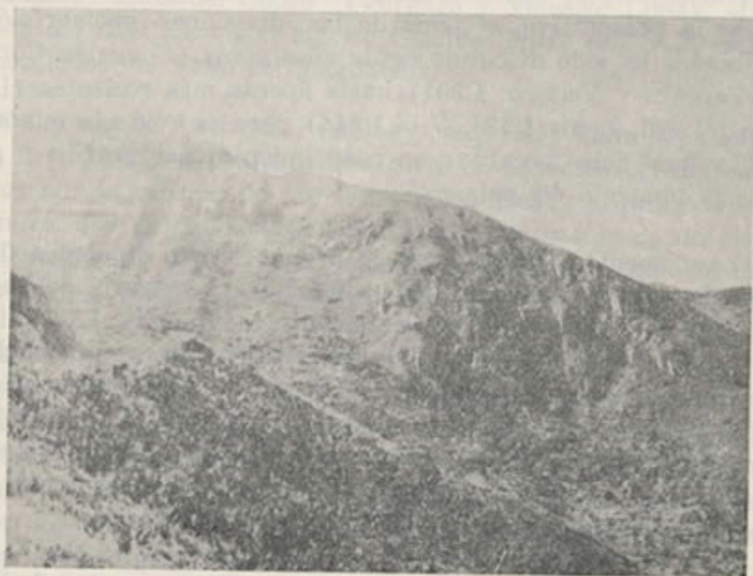
Fig. 3. Rocas desnudas en las pendientes de Matasano. Carretera Medellín-Yarumal
