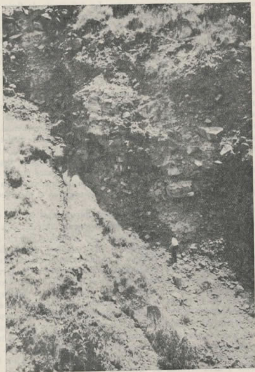
Fig. 12 - Taludes - Quebrada al Este de Bello
